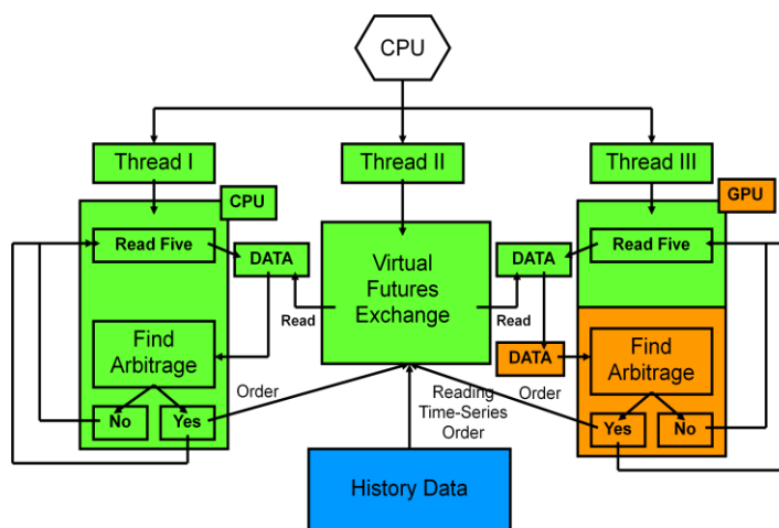
圖4 虛擬交易平台
