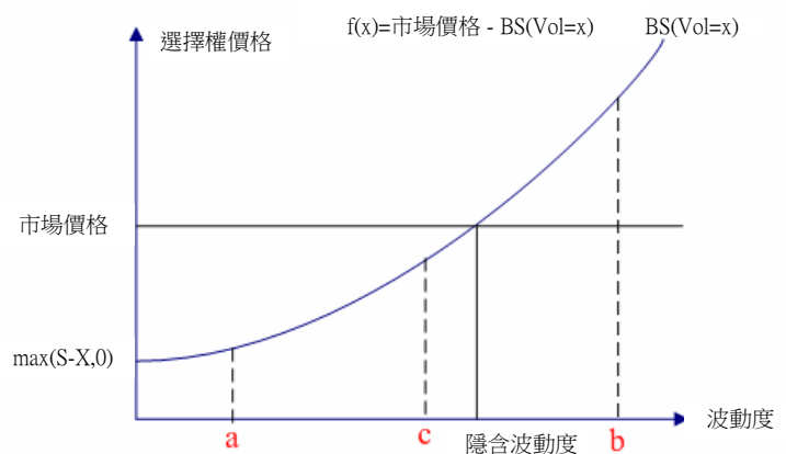
圖 5 二分法計算 資料來源：戴天時(2005) C++ 財務程式設
