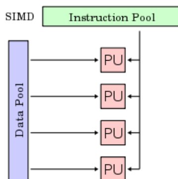
圖3 SIMD平行運算架構
