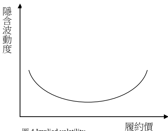
圖 4 Implied volatility smile
